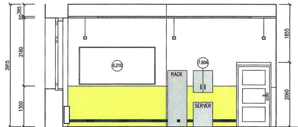
POHLED D-D' 1:50
