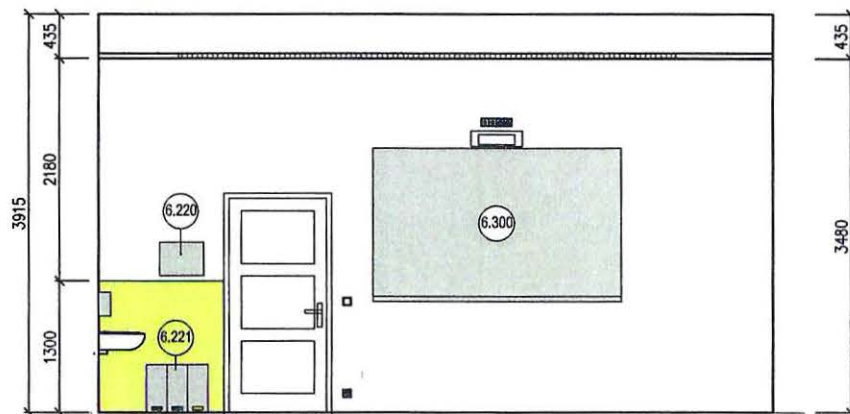
POHLED B-B' 1:50
