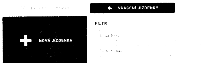
Obrázek 6 - Nová jízdenka
