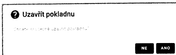
Obrázek 4 - Uzavřít pokladnu
