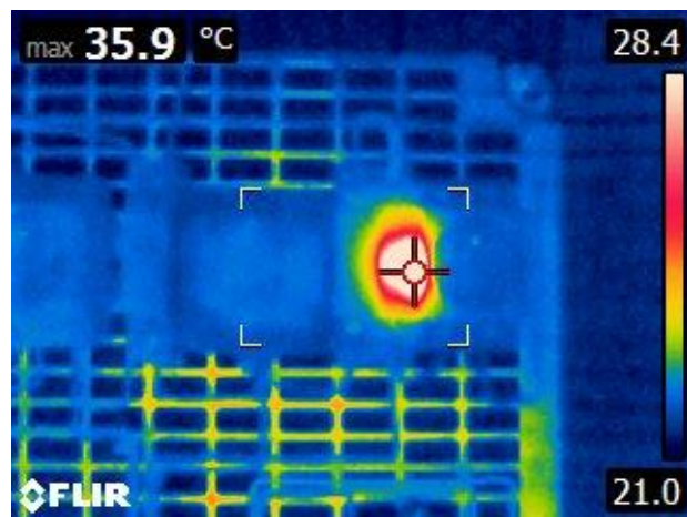
bez funkce MSX (běžné termokamery)
