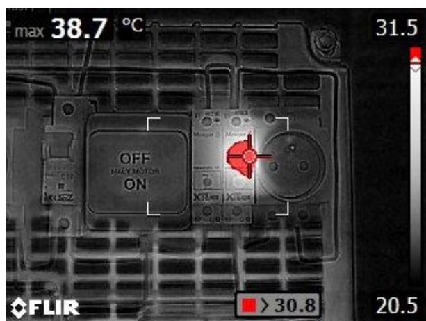
Funkce izoterma s funkcí MSX
