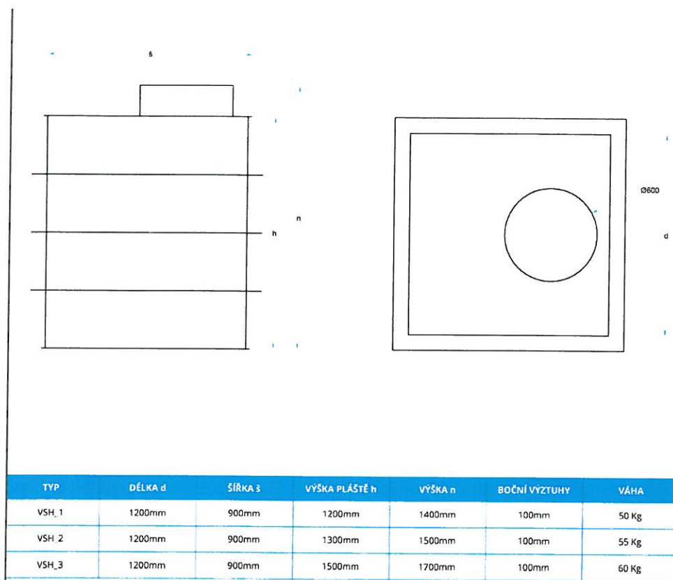
Obrázek 2a Specifikace vodoměrné šachty
