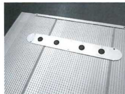
OAE060 - 4-tlačítkové nášlapné kontakty na plošině
