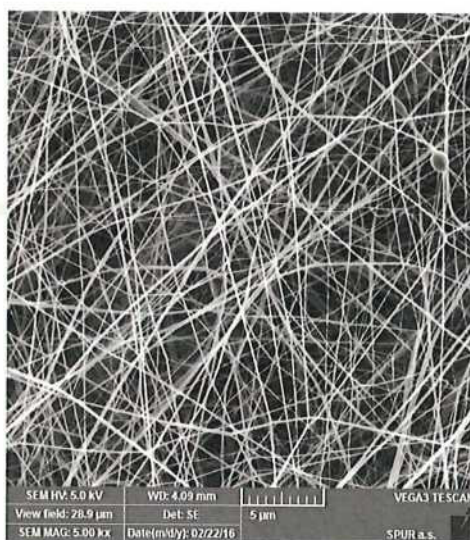
Typická nanostruktura filtračního materiálu SpurTex® VS L2 V1 (zvětšeno 5000krát na elektronovém mikroskopu).
