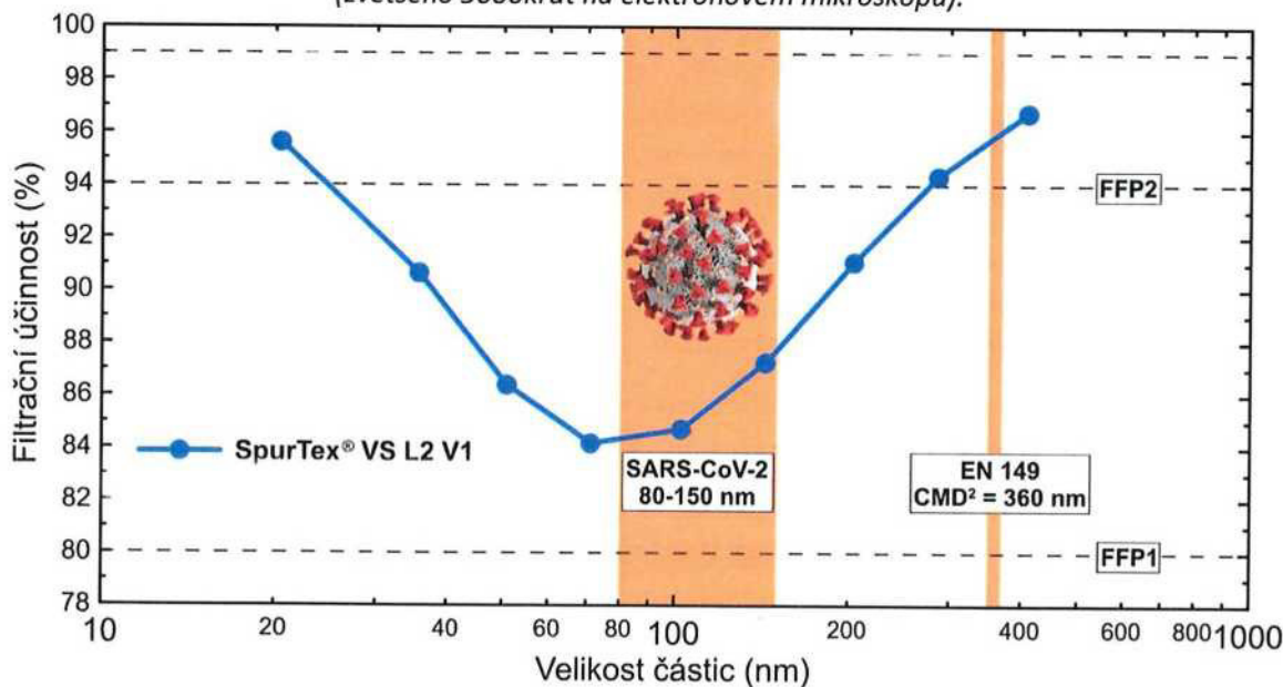
Filtrační účinnost materiálu SpurTex® VS L2 V1 při průtoku vzduchu 30 l.min -1 .
