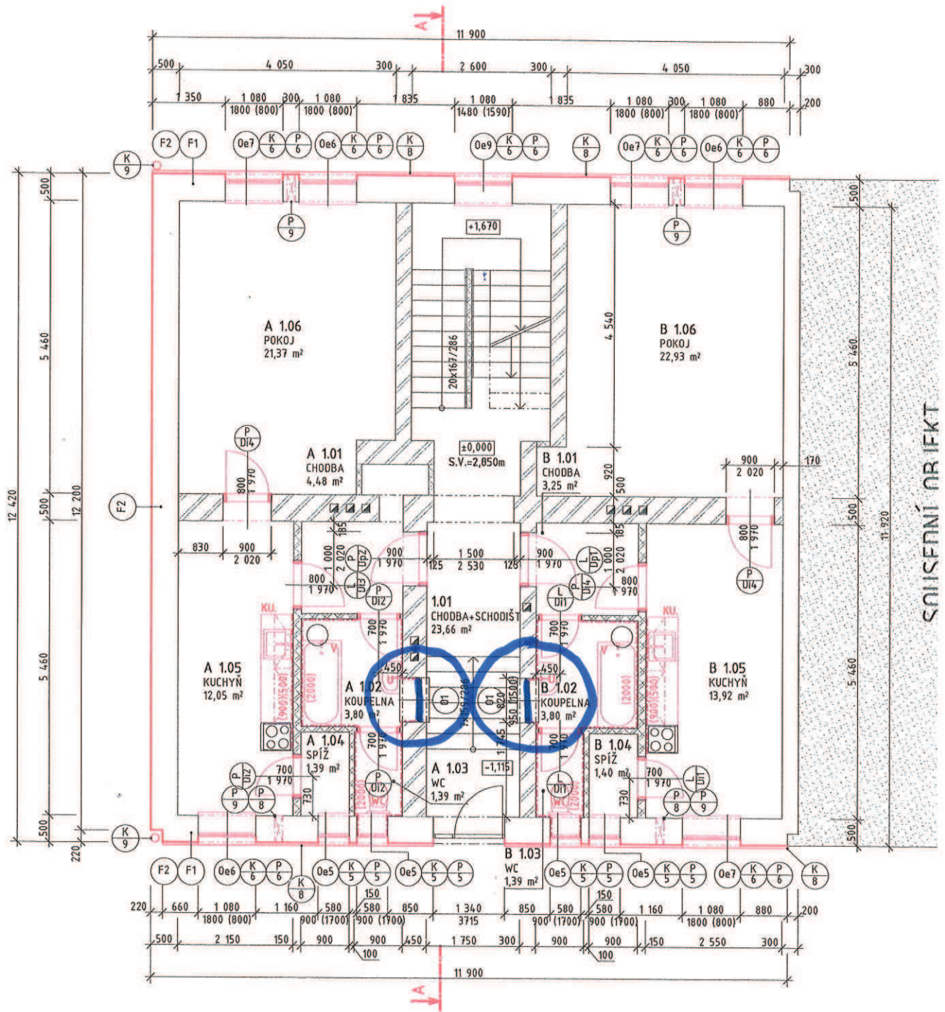
Tabulka místností 1.NP
