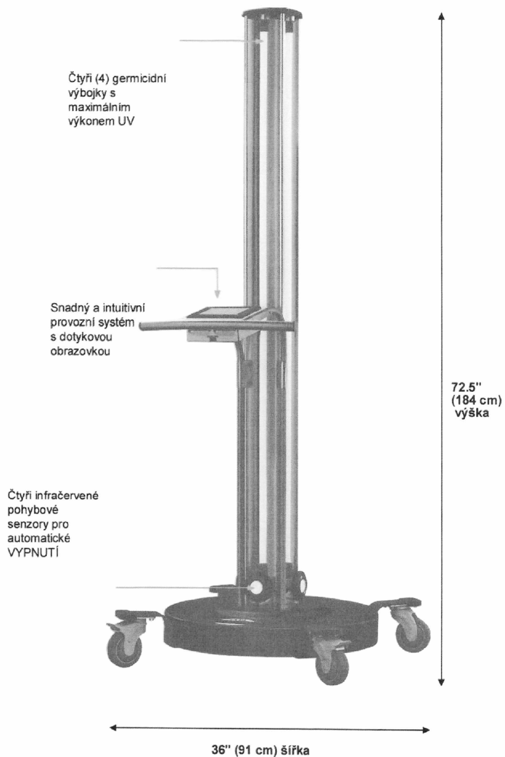
Obrázek 1: UVDI-360 systém
