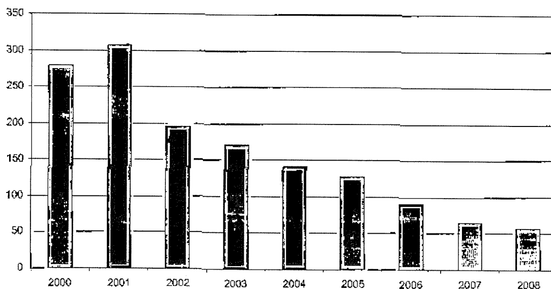
Produkce kapalných RAO z bloků 1 a 2 (m 3 )
