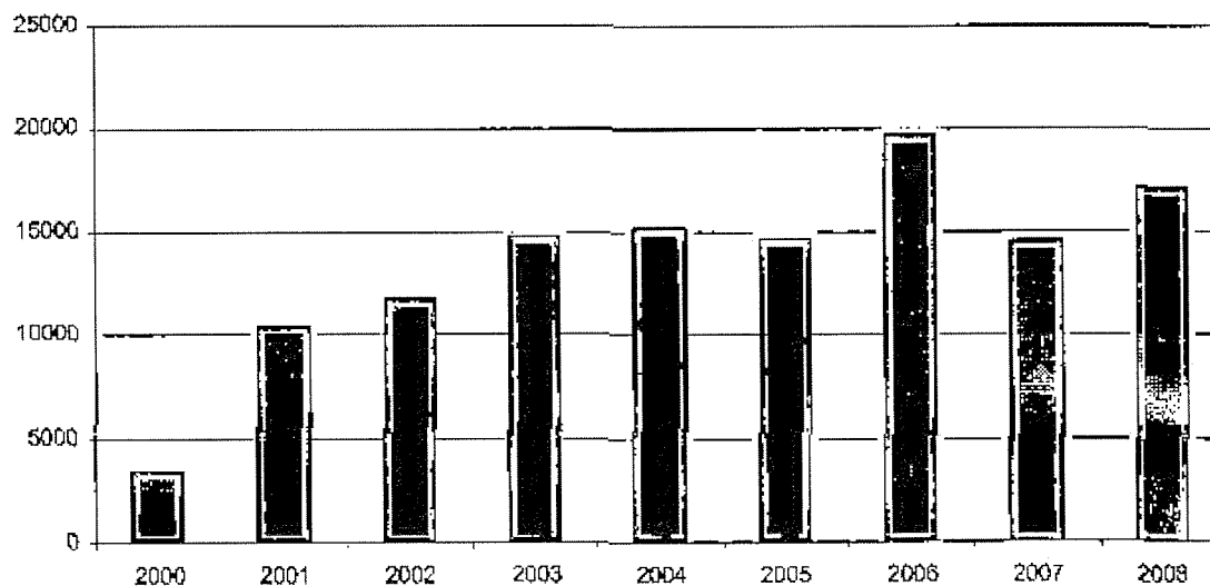
Produkce pevného radioaktivního odpadu vzniklých při provozu bloků 1 a 2 v letech 2000 až 2008 [kg]
