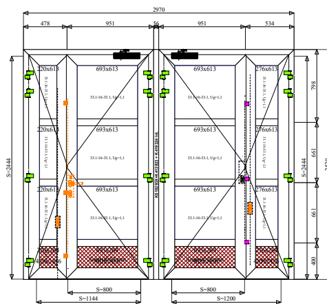
VNĚJŠÍ POHLED
