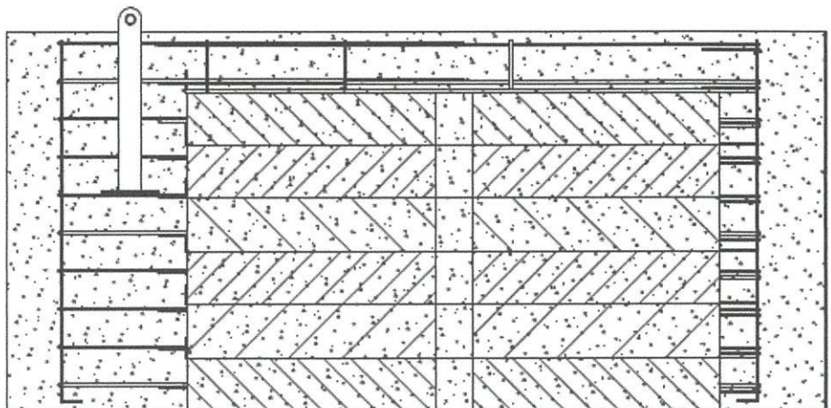
Obrázek 2: Kotevní blok sloupu SL01
