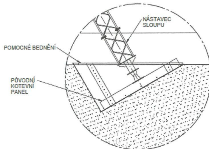
Obrázek 1: Řešení patky sloupu
