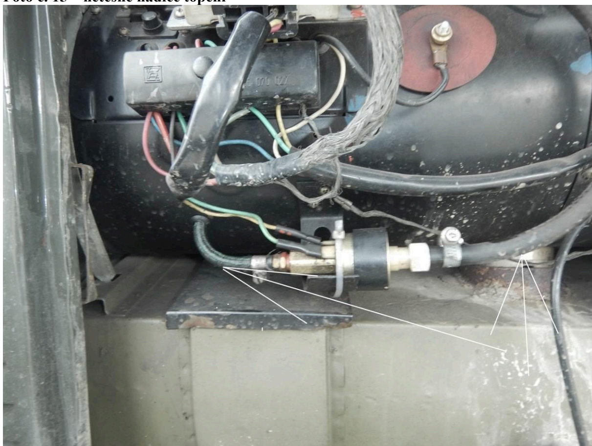
Foto č. 15 – netěsné hadice topení
