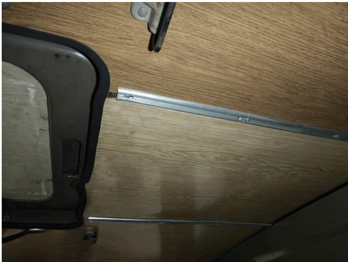
Foto č. 14 – netěsnost pot hledáčkem kabiny
