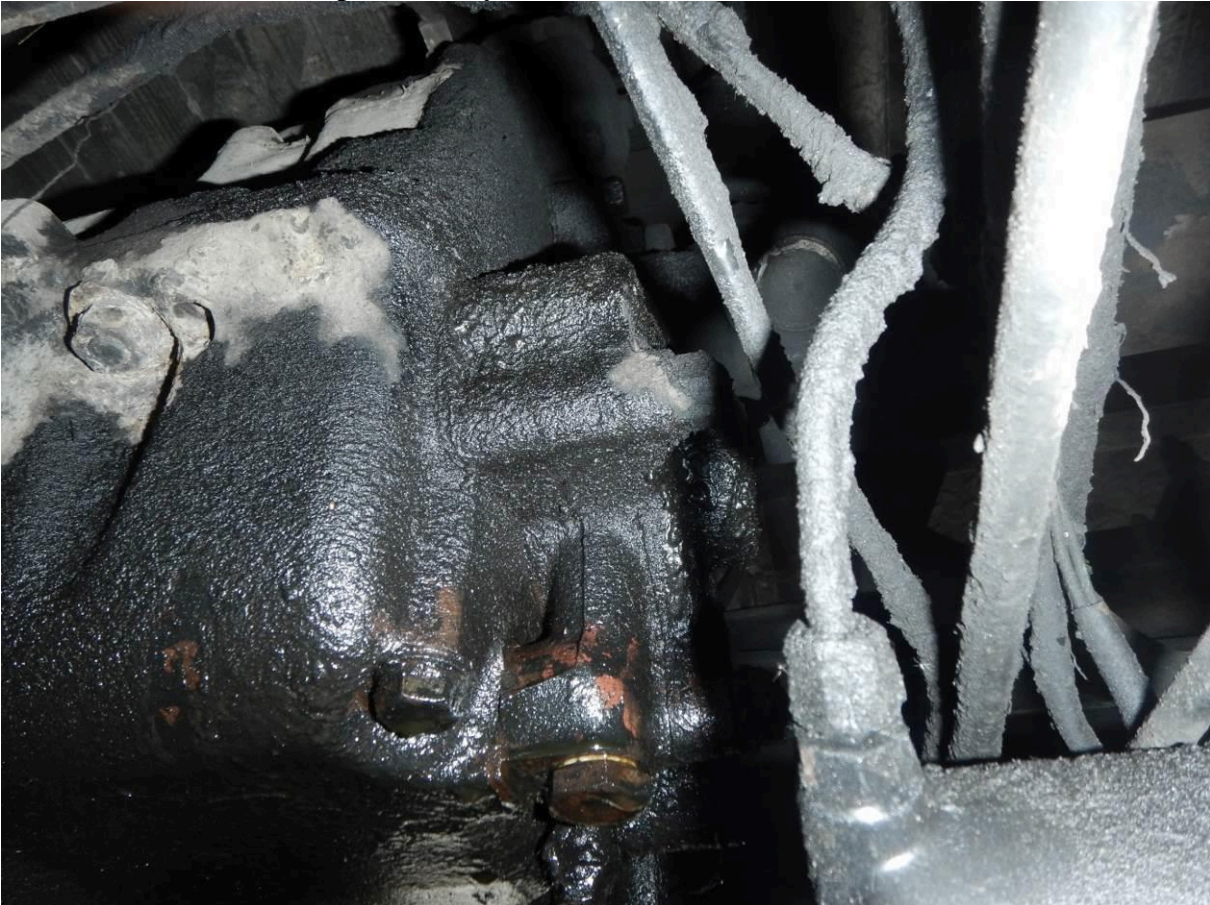
Foto č.8 – netěsnost čela převodovky
