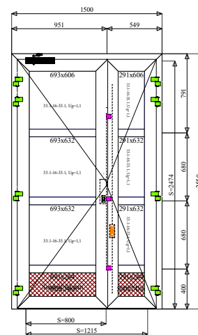
VNĚJŠÍ POHLED
