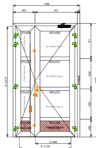
VNĚJŠÍ POHLED
