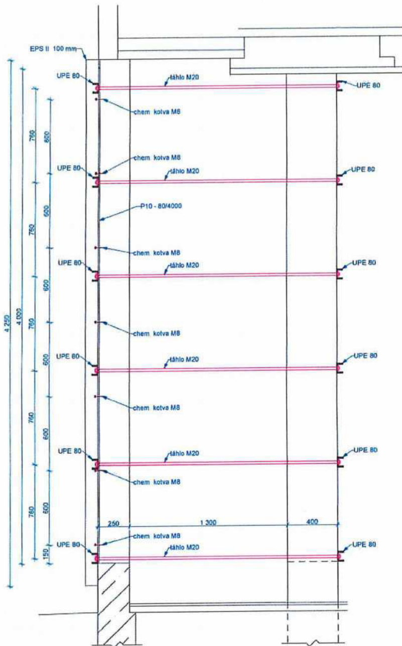
POHLED A - A; M 1:20
