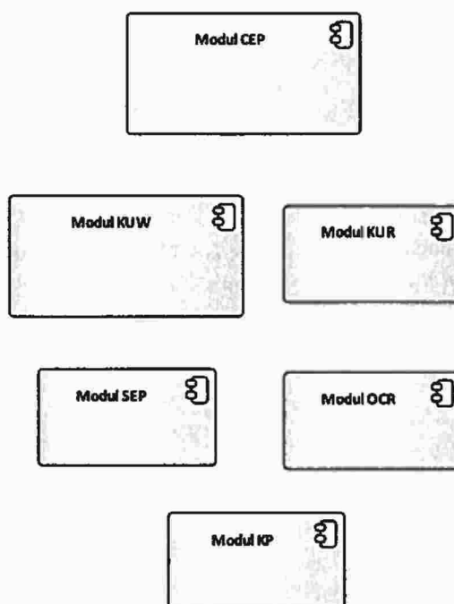
Obrázek 5 – Sharepoint diagram
