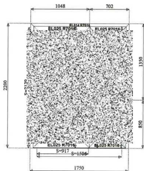
Poz. 1b: Hliníkové dveře 1750 x 2200mm:- 4ks VENKOVNÍ POHLED
