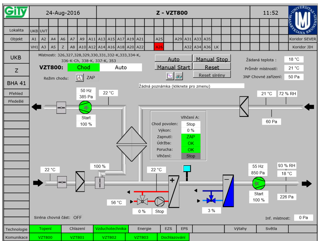
Obrázek 3.1: Obrazovka technologie
