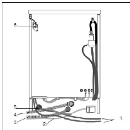
Obrázek 2.3 Zadní část jednotky
