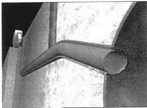
- zavedení impregnovaného rukávce do rekonstruovaného úseku a jeho vytvrzení
