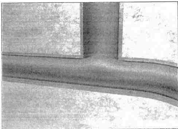
- prořezání stávajících zaústěných přípojek robotem
