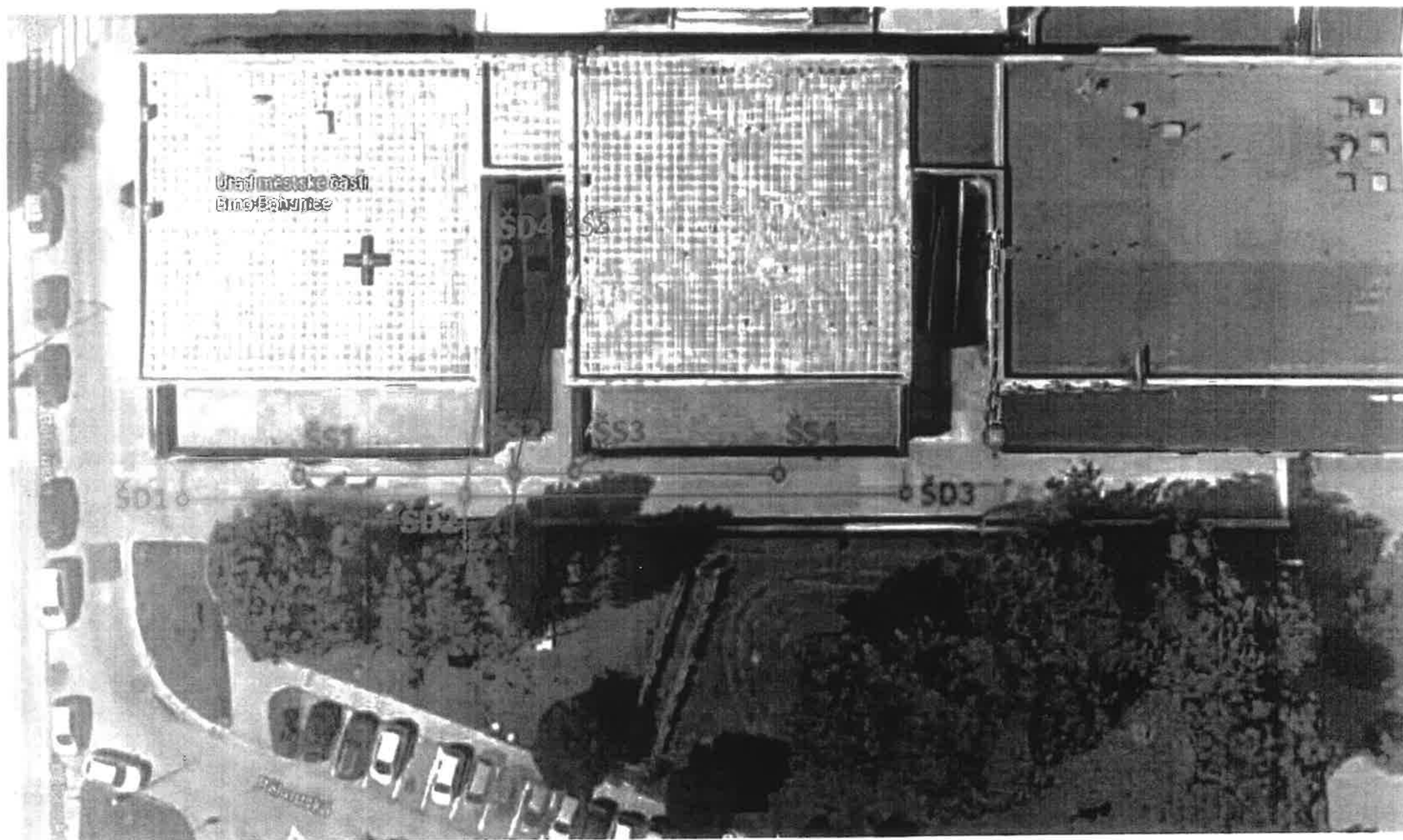
Nákres kanalizačních přípojek pro objekt ÚMČ Brno-Bohunice
