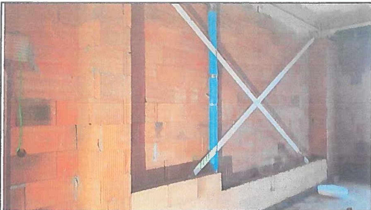
Oboustranné obezdění táhel ocelové kce.
