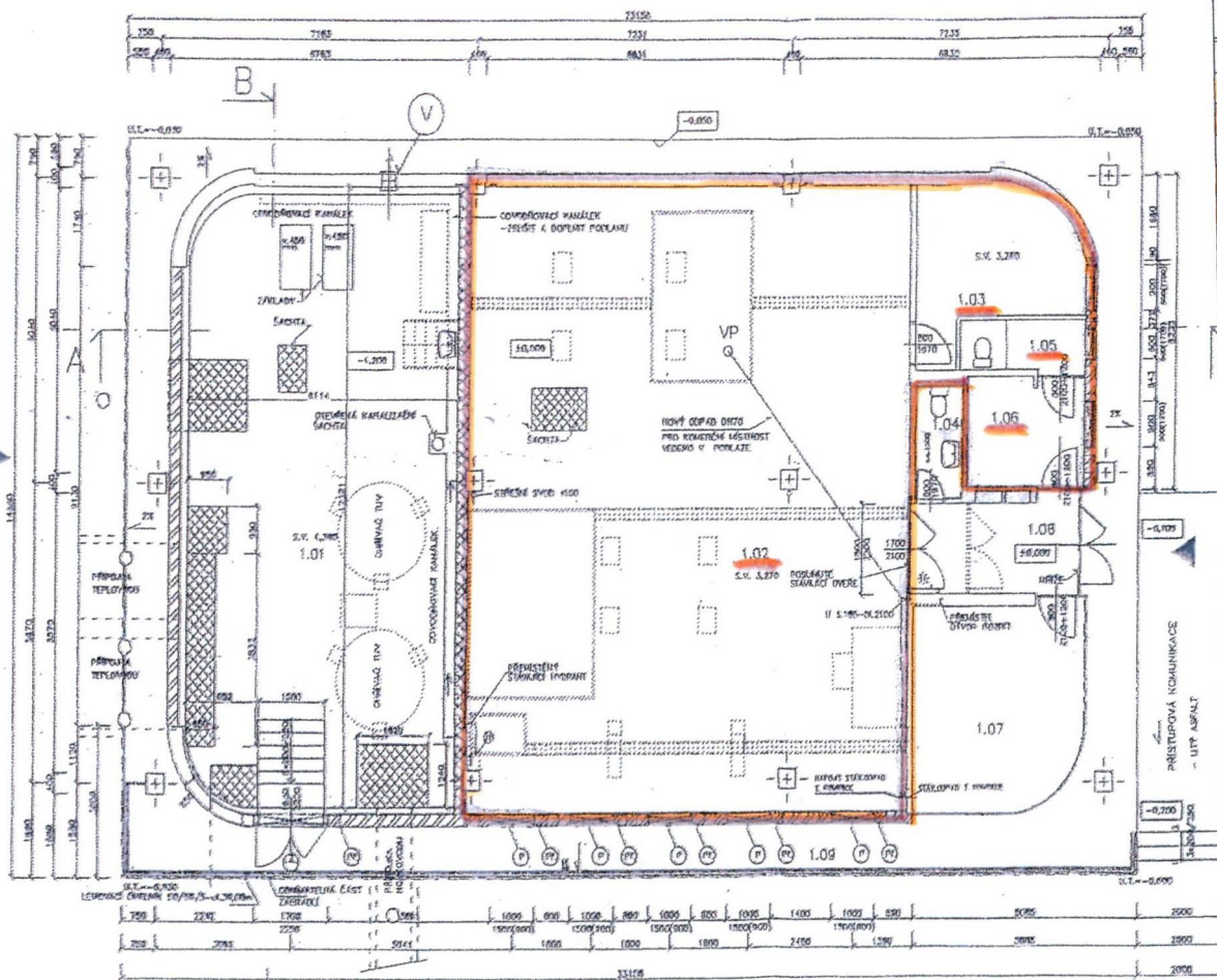
PŮDORYS VÝMĚNIKOVÉ STANICE VS 14 M 1:50 BRNO-LÍŠEŇ NOVÝ STAV
