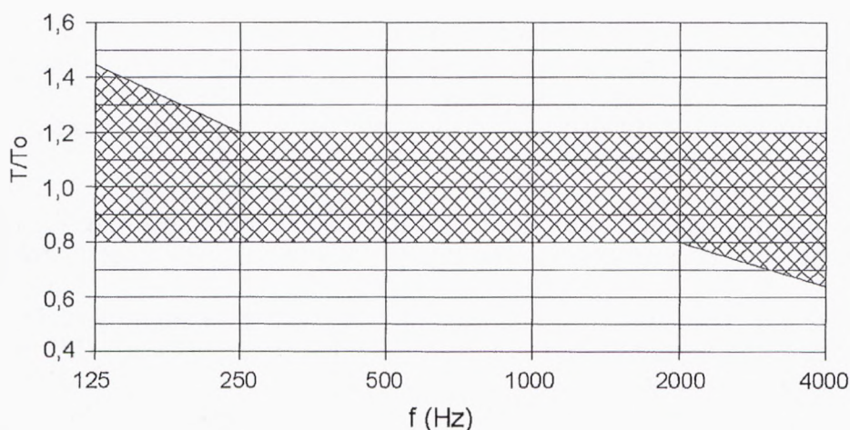
Obr. 1 - ČSN 73 0526 - Přípustné rozmezí poměru dob dozvuku T/T_0 obsazeného prostoru určeného k přednesu hudby i řeči v závislosti na středním kmitočtu oktávového pásma
