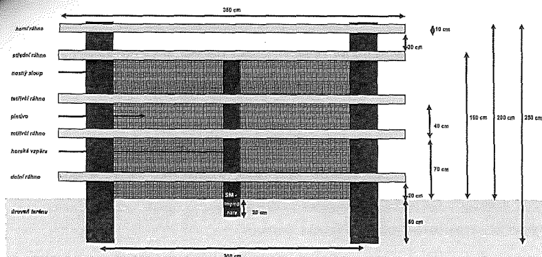
Návrh jednoho pole horské oplocenky (bez zavětrovacích vzpěr):
