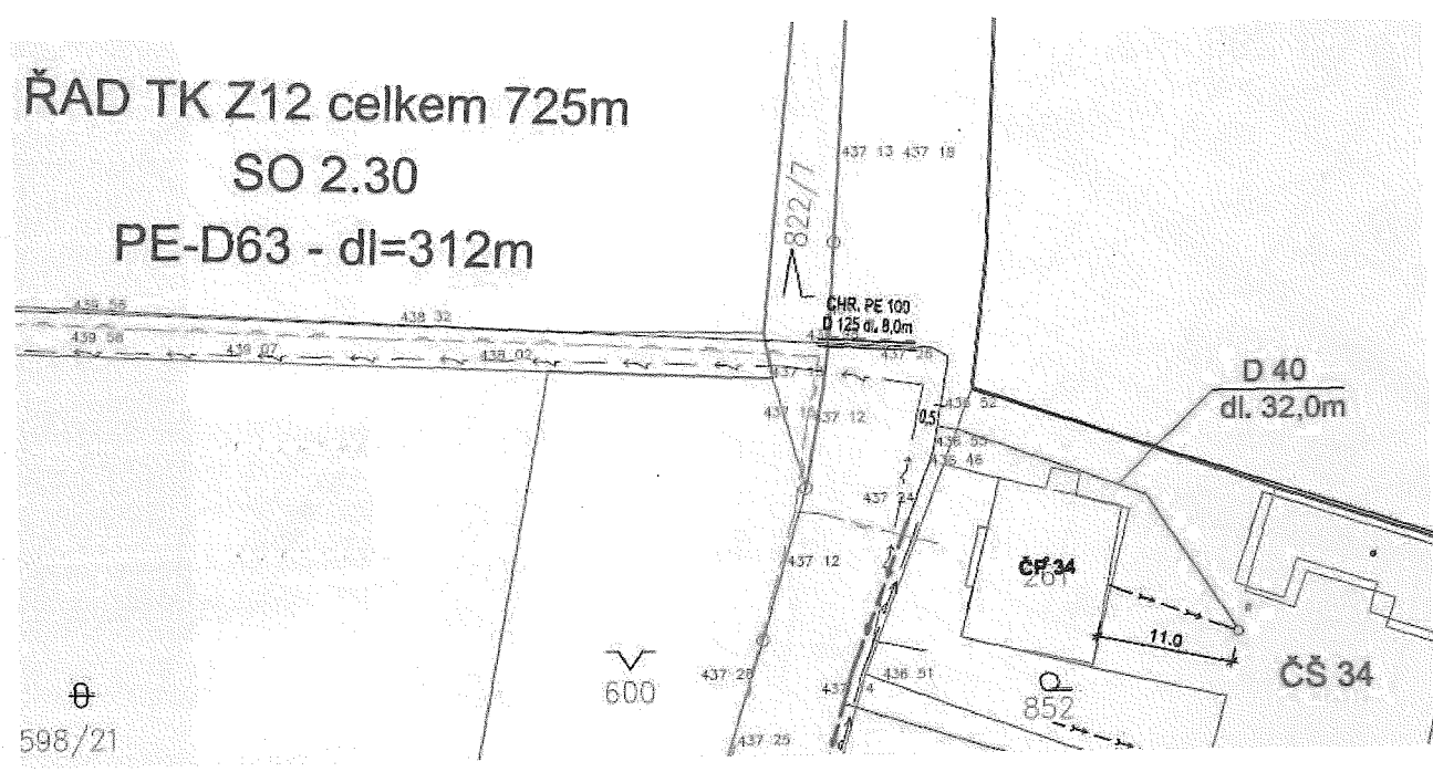
Suchovod tlakové kanalizace řad TK Z12 – p.č. 822/7 – s vodovodem
