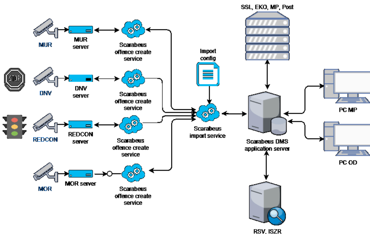
OBRÁZEK 1 BLOKOVÉ SCHÉMA KOMUNIKACE
