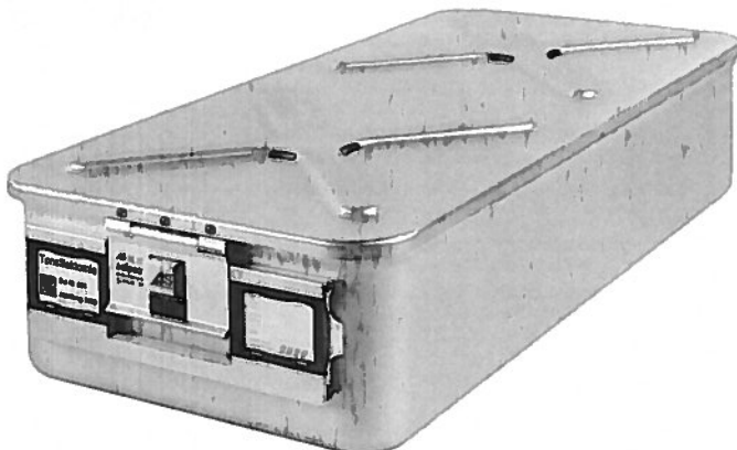
Sterilizační kontejner (587x279x131mm)
