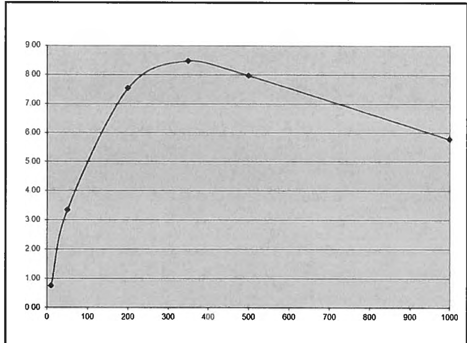
Obrázek 8 – Výstupní výkon diatermie (100% nastavení)
