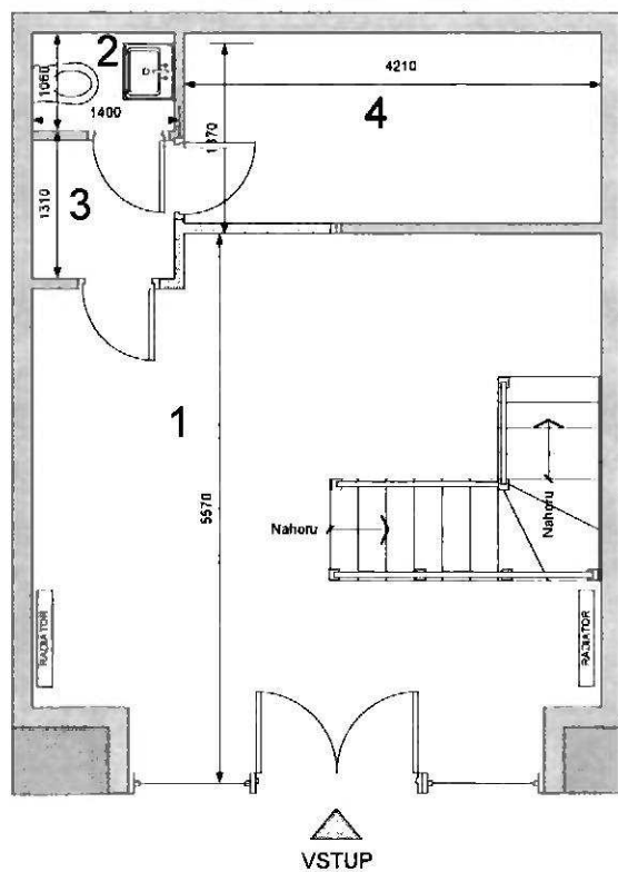
1.NP
