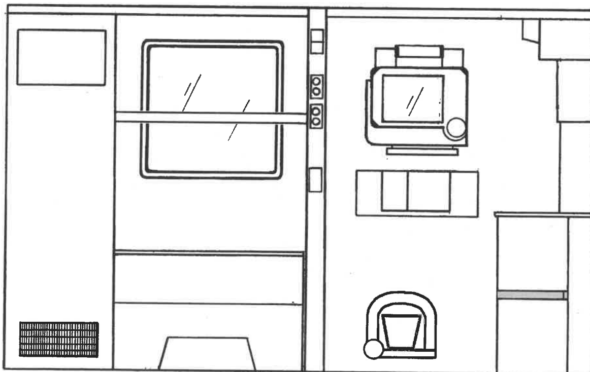
Schéma nábytkové zástavby vozidla - levý bok:
