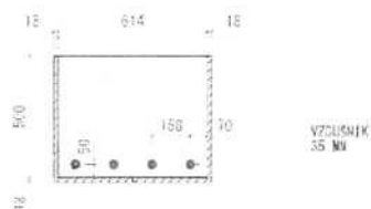
ŘEZ C-C
