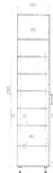
ŘEZ B-B
