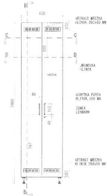
NÁRYS
