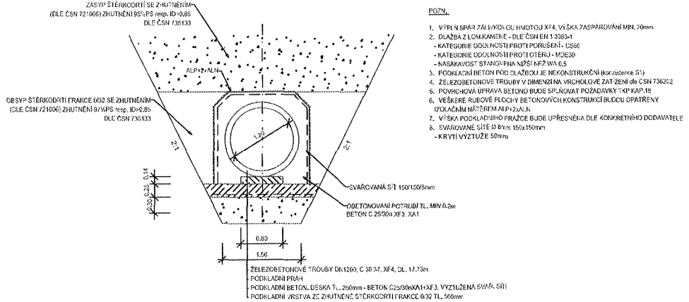
SCHÉMA ULOŽENÍ POTRUBÍ M 1:50
