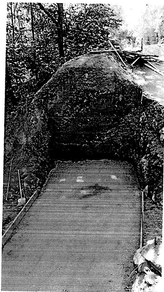
SO 104 – Zásyp ŠD fr. 0-32mm tl.= 0,5m pod základ (povodní strana)
