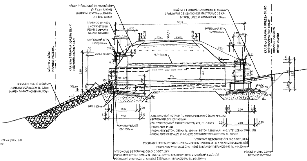
SCHÉMA ULOŽENÍ POTRUBÍ M 1:50
