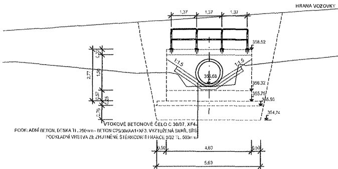
POHLED NA VTOK
