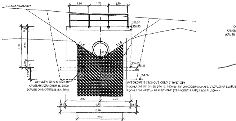
POHLED NA VÝTOK
