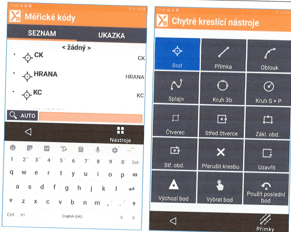
Obrázek 4 - snadné kódování a inteligentní kreslení situace přímo při měření
