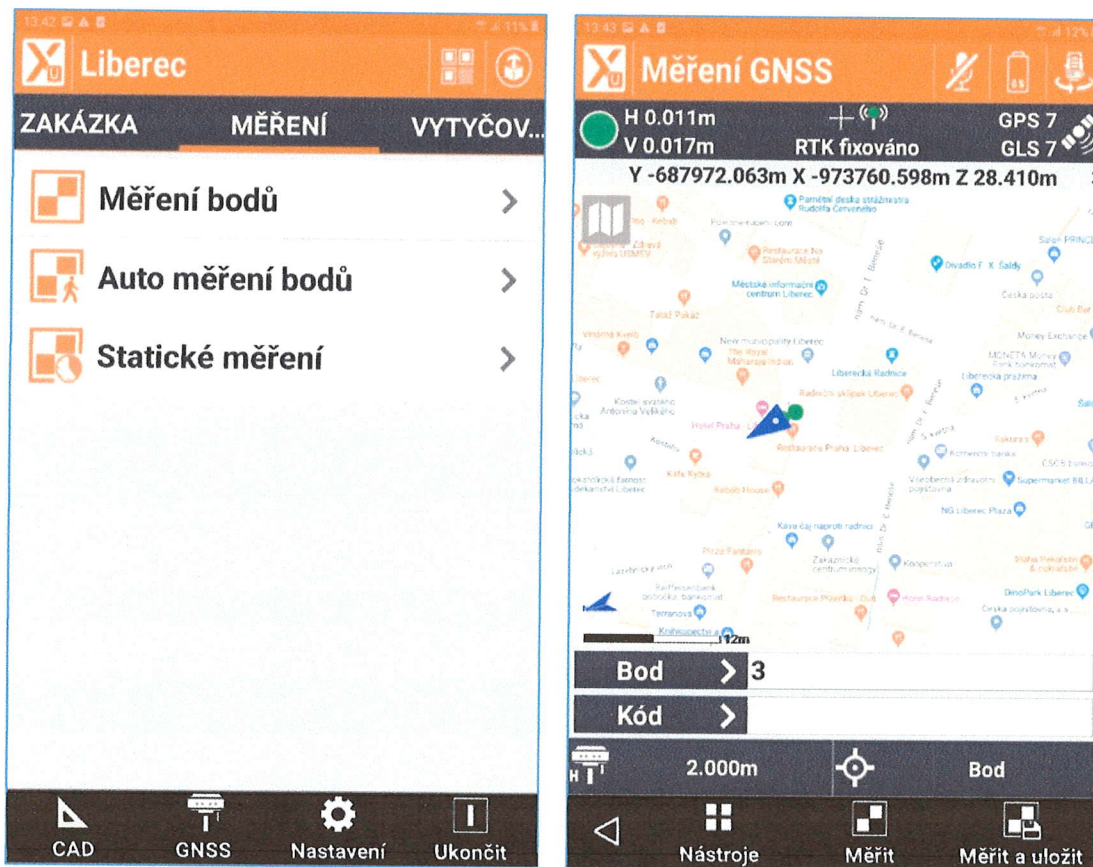
Obrázek 2 - vstup do měření, měření s podkladem GoogleMaps
