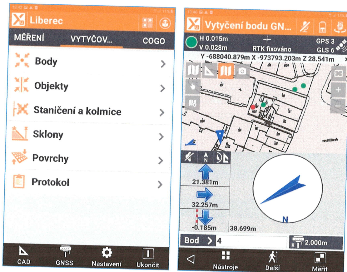
Obrázek 5 – možnost vytyčování bodů i objektů, obrazovka při vytyčování
