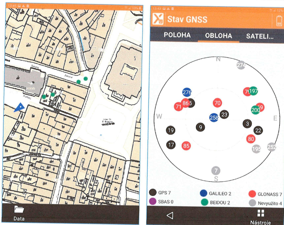
Obrázek 6 – komplexní informace o měření i o aktuálním stavu satelitů
