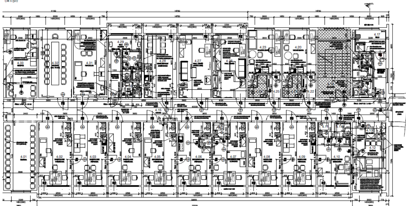
PŮDORYS 4.NP - nový stav (M 1:50)
