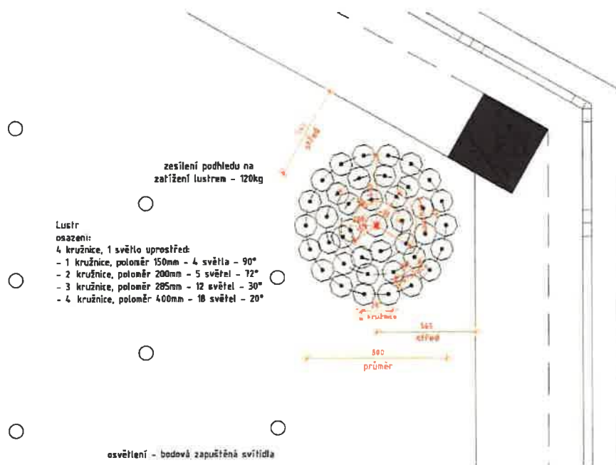
schematický půdorys
