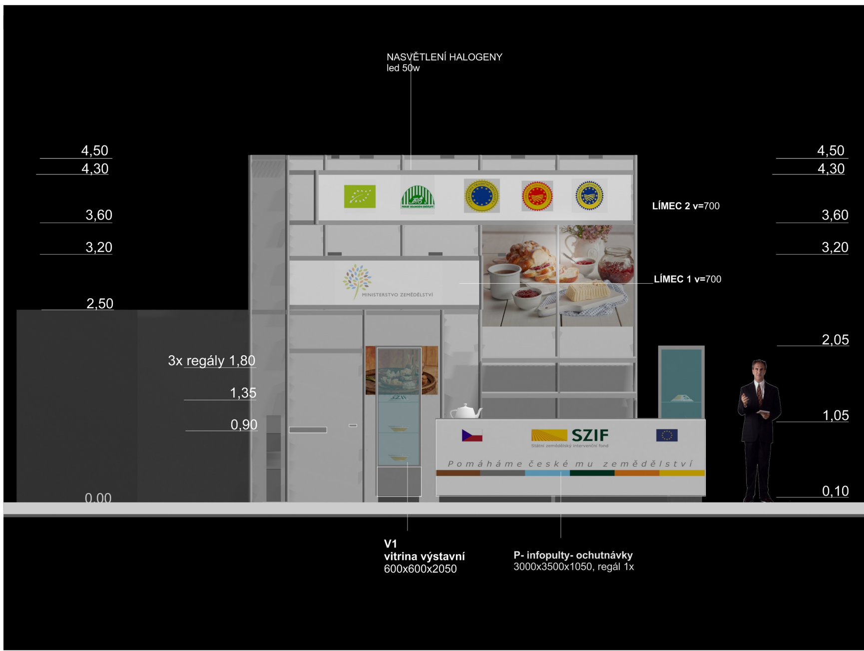
pohled čelní 1_50
