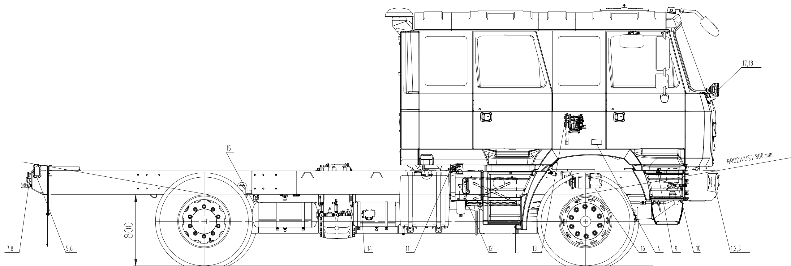
SEZNAM ELEKTRICKÝCH A ELEKTRONICKÝCH ZAŘÍZENÍ PODVOZKU TATRA POD ČÁROU BRODĚNÍ
