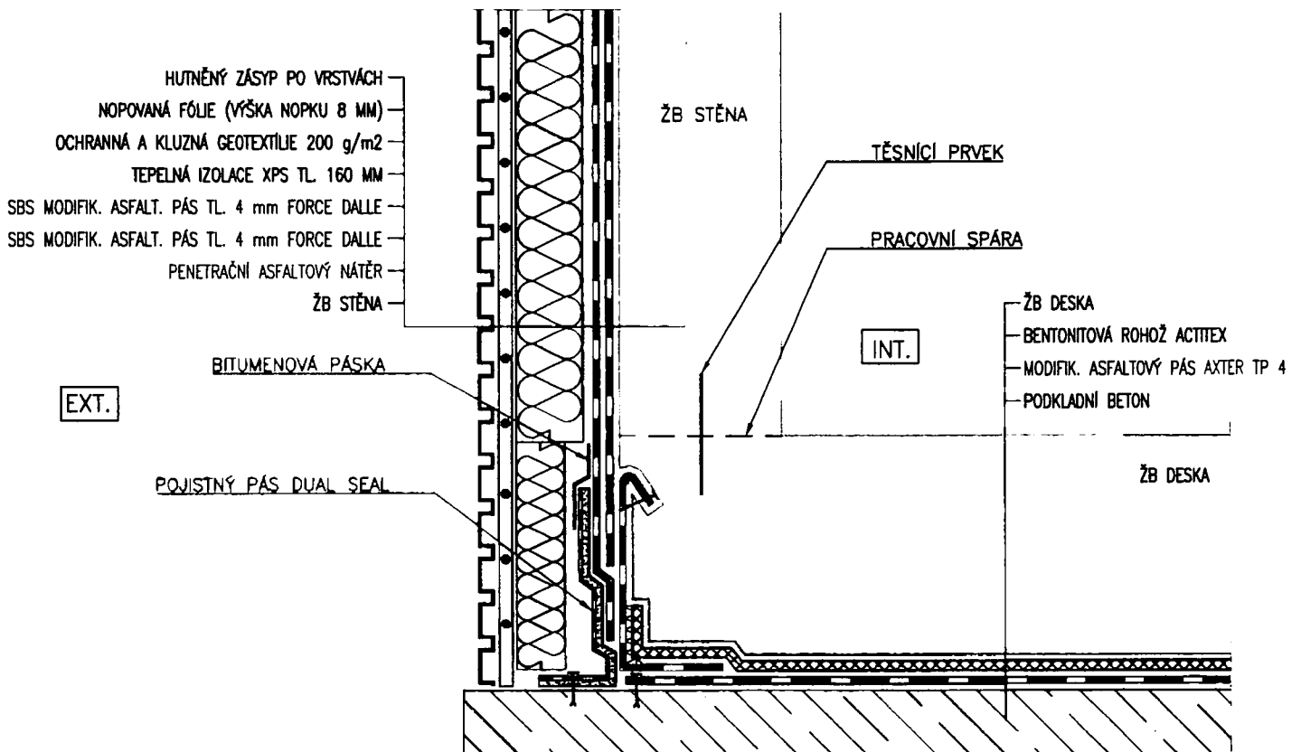
SO.01 SVISLÝ ŘEZ ZÁKLADOVOU DESKOU A STĚNOU
