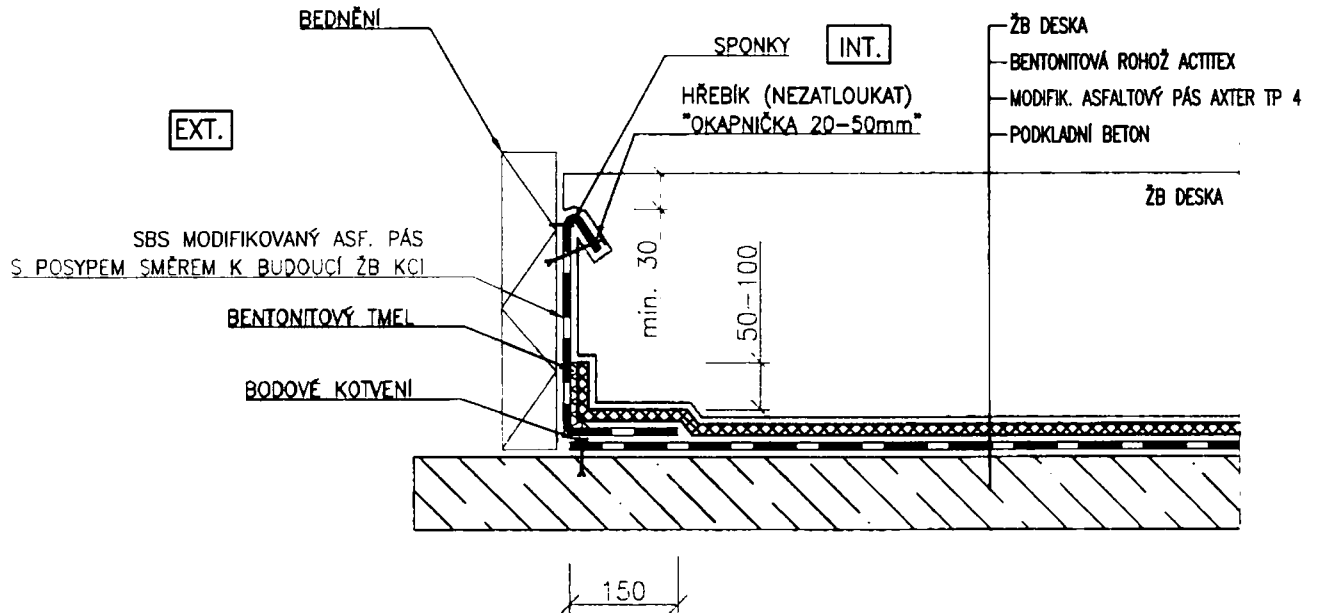
SO.01 SVISLÝ ŘEZ ZÁKLADOVOU DESKOU A STĚNOU
