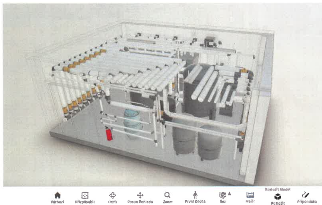
Obr. 4 Stejný BIM model technické místnosti v areálu AdMaS (VUT) ve webové aplikaci společnosti Autodesk
