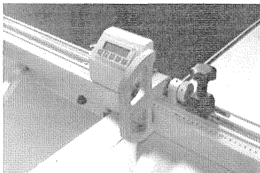
Obr. Digitální odečet pravítka
