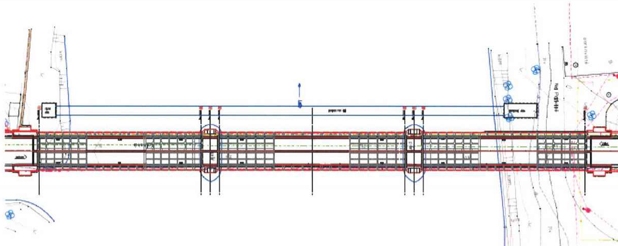
Obrázek 1 – Situace mostu a předpokládaného umístění kolektoru
