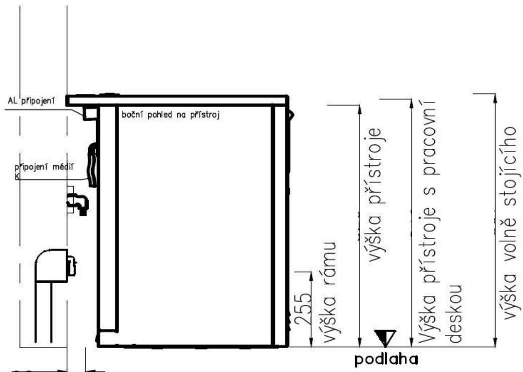
Boční pohled
