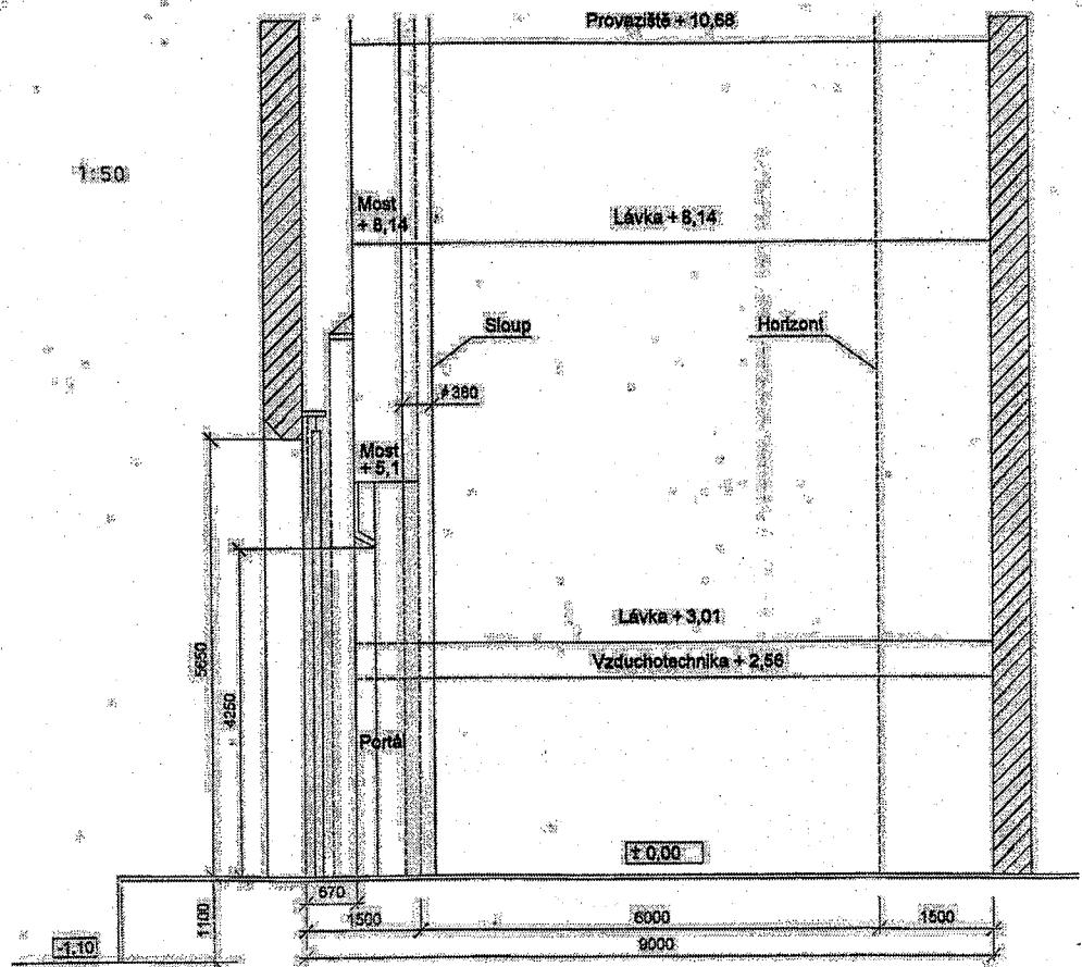
Řez jeviště:
