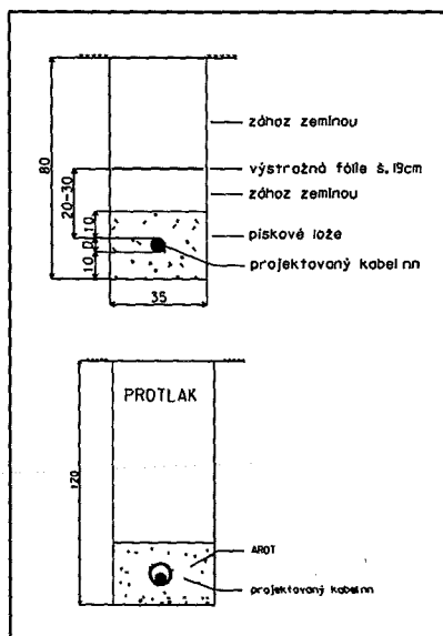
Řezy kabelovou trasou
