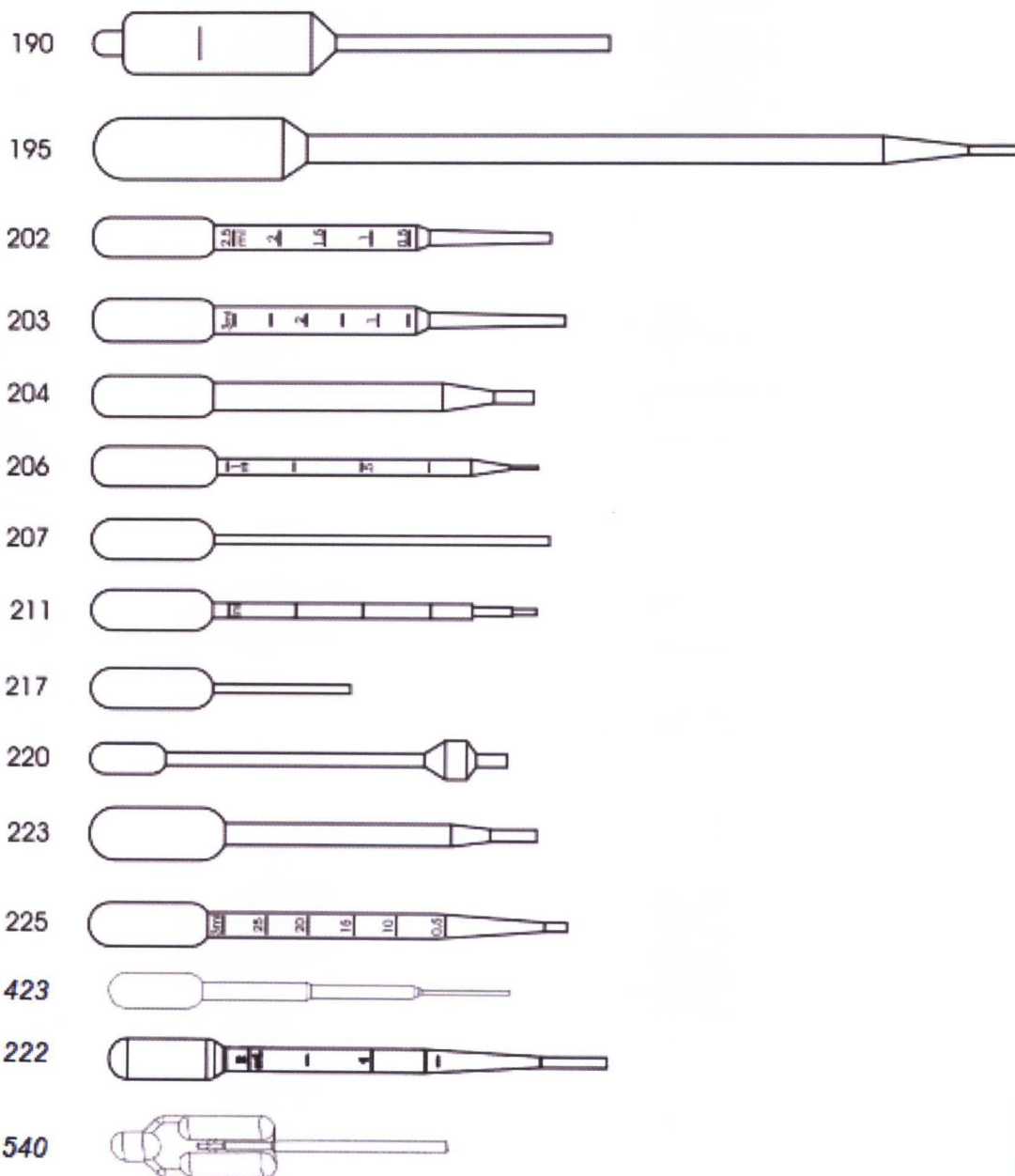
Obrázek 1 - Pasteurovy pipety nesterilní
