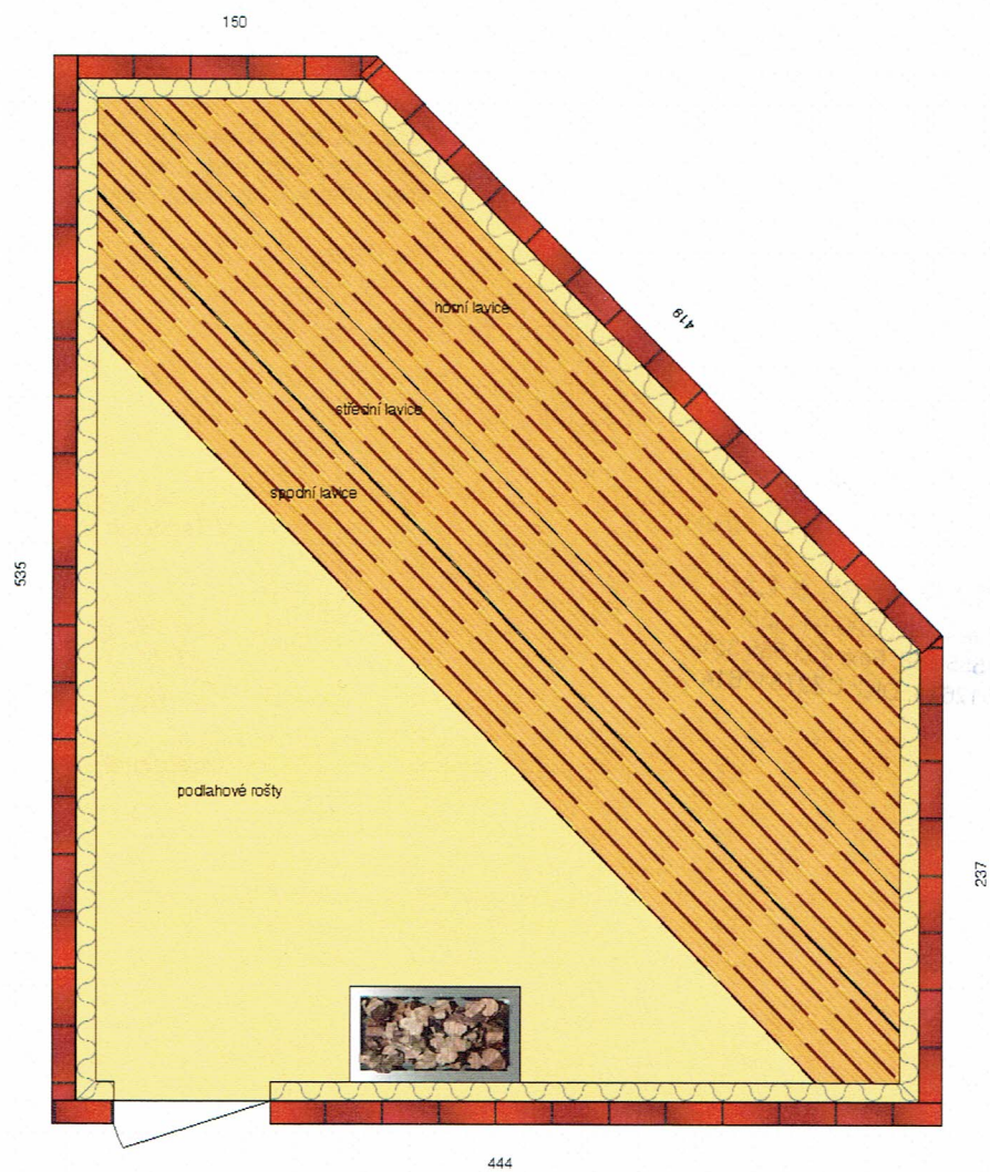
Příloha č. 1) půdorys saunové kabiny
