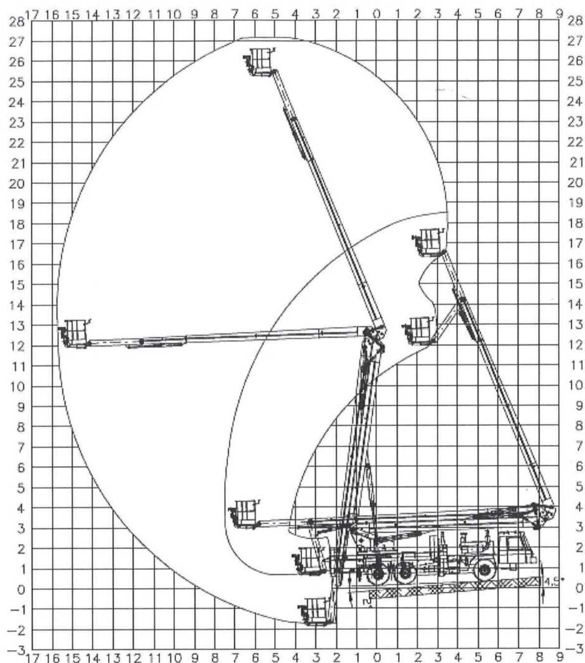
Pracovní diagram
