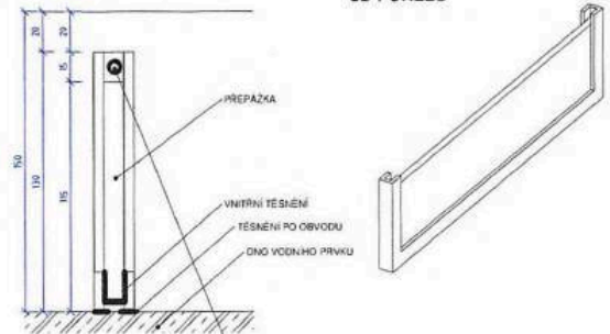
3D POHLED
