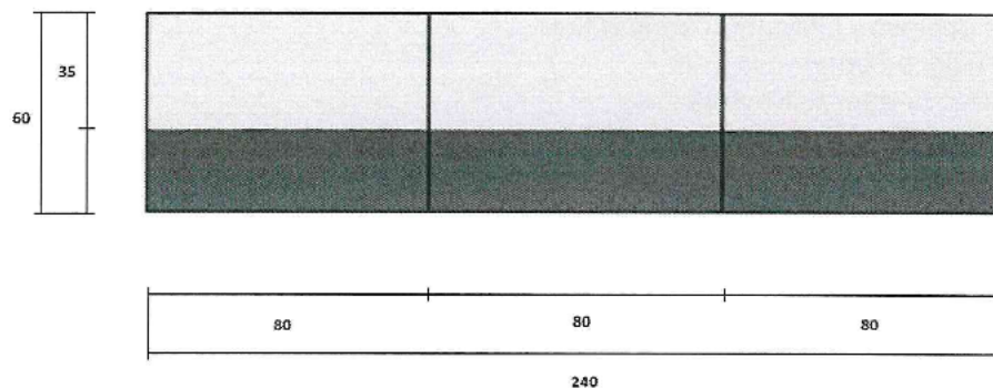
pohled shora
