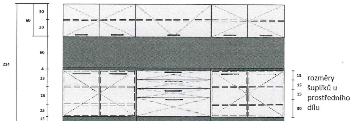
čelní pohled
