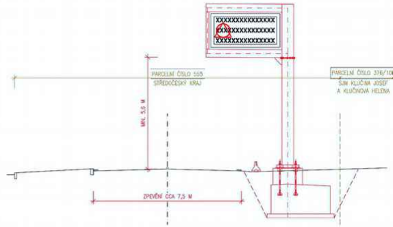
VZOROVÝ PŘÍČNÝ ŘEZ 1:100 (PROTI SMĚRU STANIČNÍ KOMUNIKACE)
