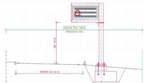
VZOROVÝ PŘÍČNÝ ŘEZ 1:100 (VE SMĚRU STANIČNÍ KOMUNIKACE)
