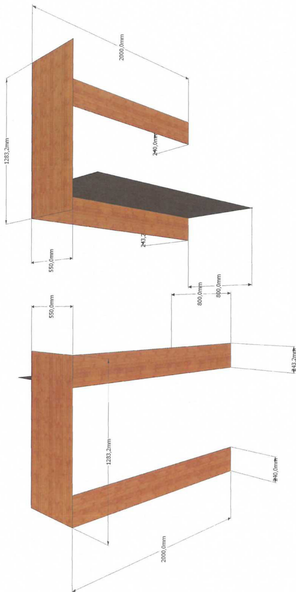
Příloha č. 5 - dveře s výztuhami V3
