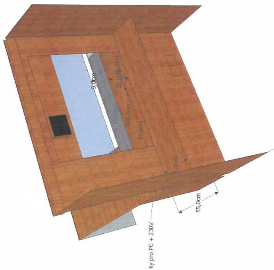
Příloha č. 3 - přepážka 160 pravá
